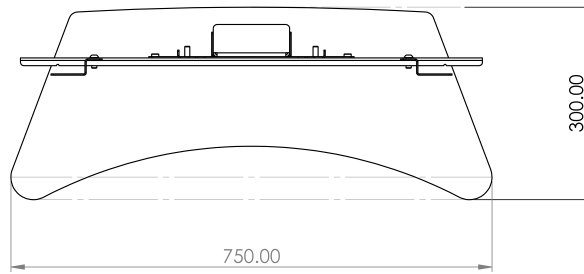
AUFSICHT (NUR STANDFUSS)
